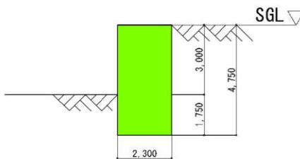
断面図
